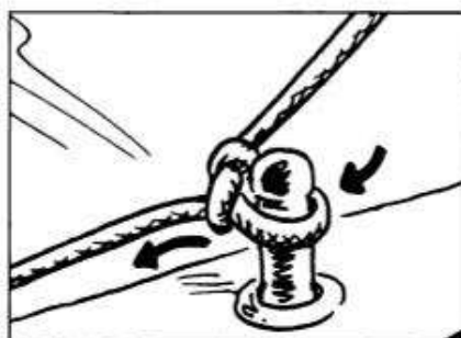
Kéo dây dầy để nút buộc siết chặt lại quanh khóa mở cửa.
