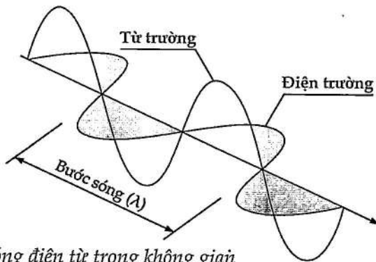
Sóng điện từ trong không gian
