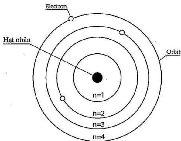
Quỹ đạo của nguyên tử
