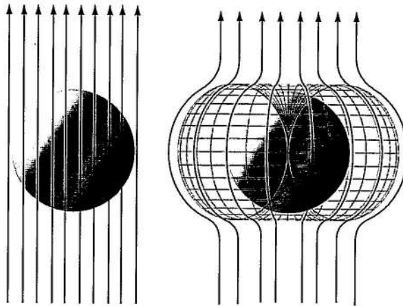
Hiện tượng khóa lượng tử tương tự với cơ chế không trọng lực của một trường năng lượng Torus
