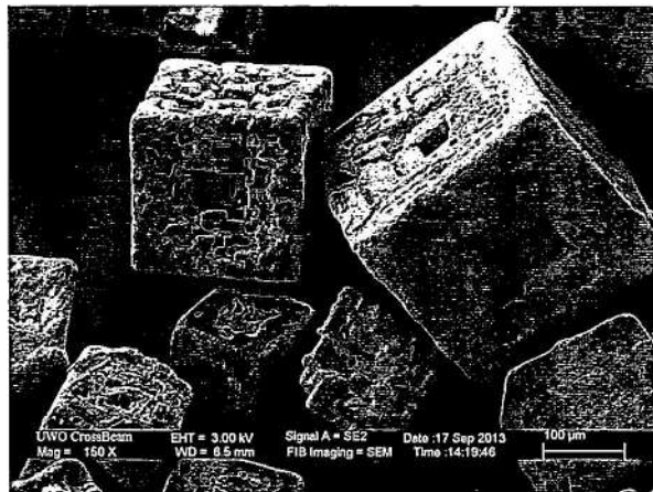
Các hạt muối nhìn dưới kính hiển vi
