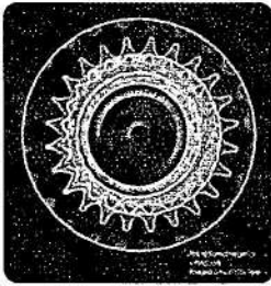
UT - 396 Hz - Antinodes: 24
