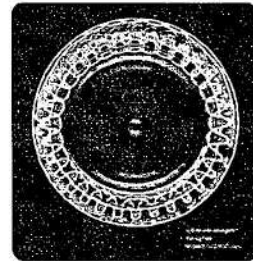
MI - 528 Hz - Antinodes: 32
